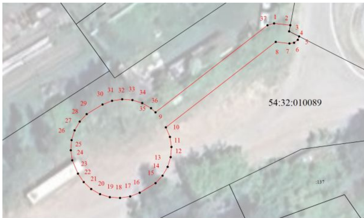
Мащтаб 1:500
